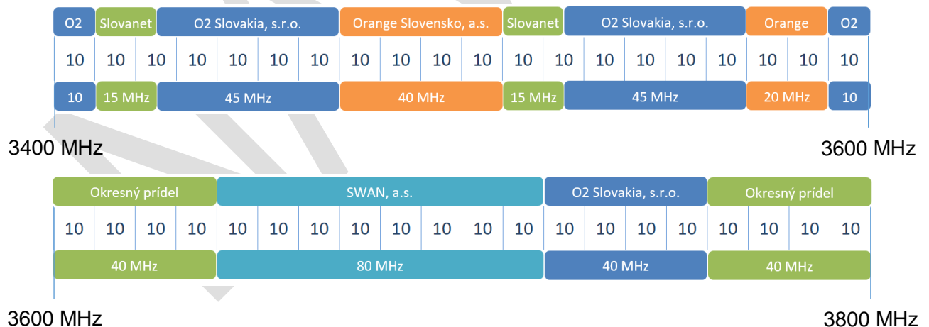
Obrázok č. 4.1: Rozdelenie frekvencií vo frekvenčnom pásme 3,6 GHz
