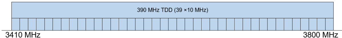
Obrázok č. 5.1: Rozdelenie frekvencií z frekvenčného pásma 3,6 GHz pre pripravované výberové konania
