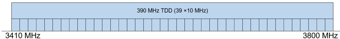
Obrázok č. 4.1: Rozdelenie frekvencií z frekvenčného pásma 3,6 GHz pre pripravované výberové konania
