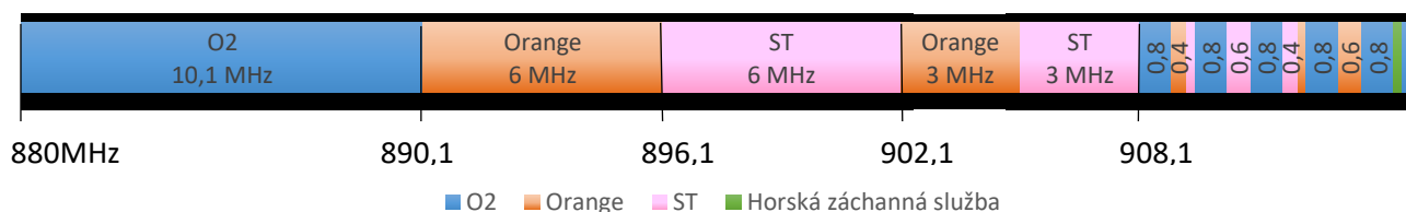
Obrázok 3.1: Rozdeľovanie frekvencií vo frekvenčnom pásme 900 MHz
