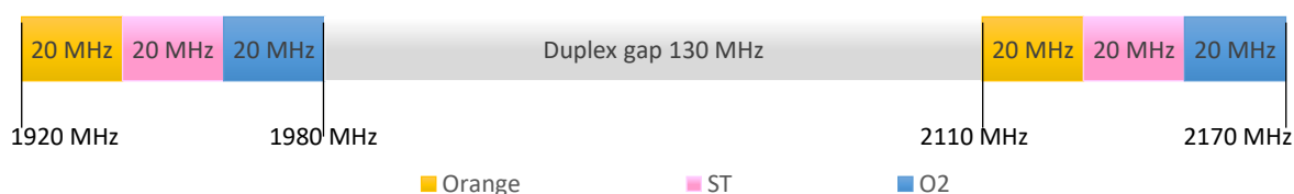
Obrázok 4.1: Rozdeľovanie frekvencií vo frekvenčnom pásme 2100 MHz
